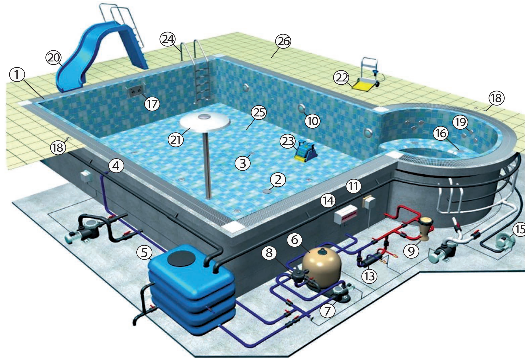
ТЕХНОЛОГИЧЕСКАЯ СХЕМА
